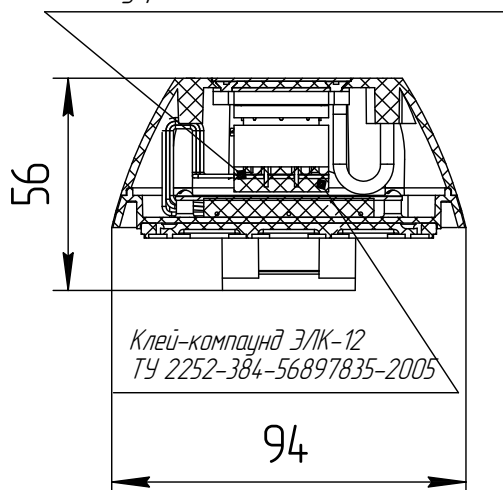
Блок управления ПР ИБЯЛ.4264.71.013
